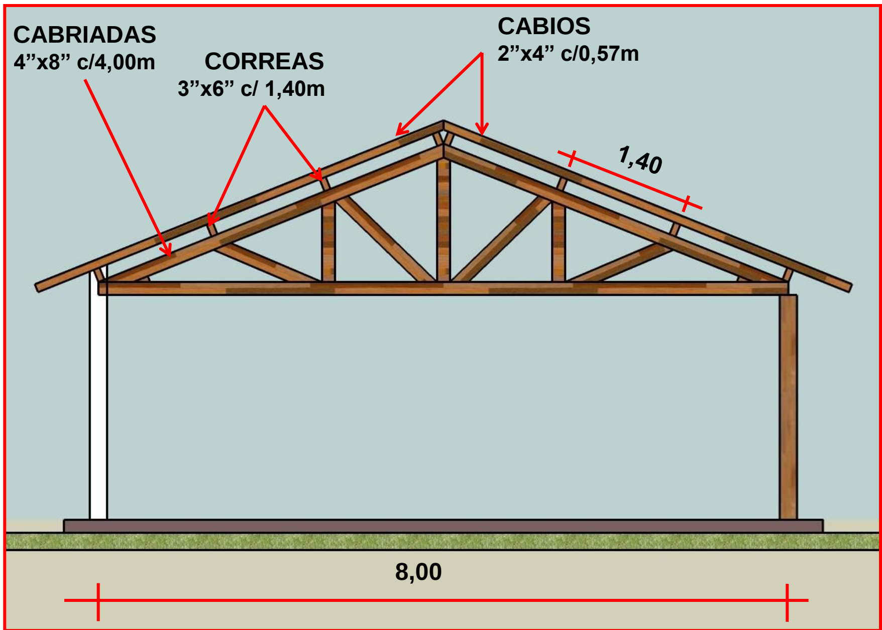
CORTE ESTRUCTURAL (Longitudinal a la pendiente)
