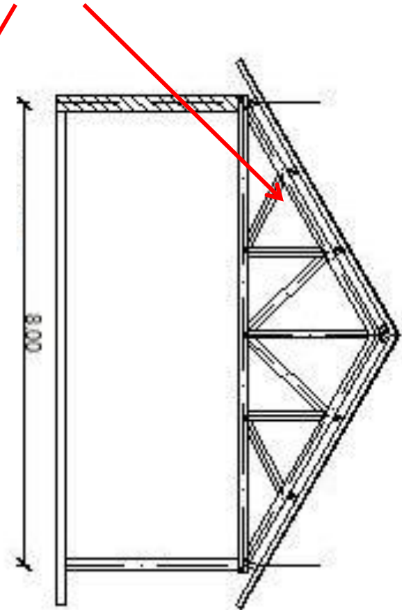
CORTE ESTRUCTURAL
